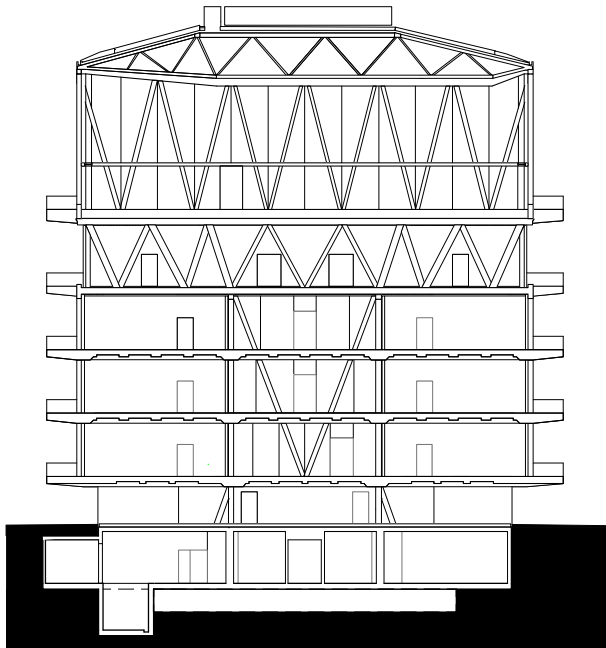
Leutschenbach, Cross Section
