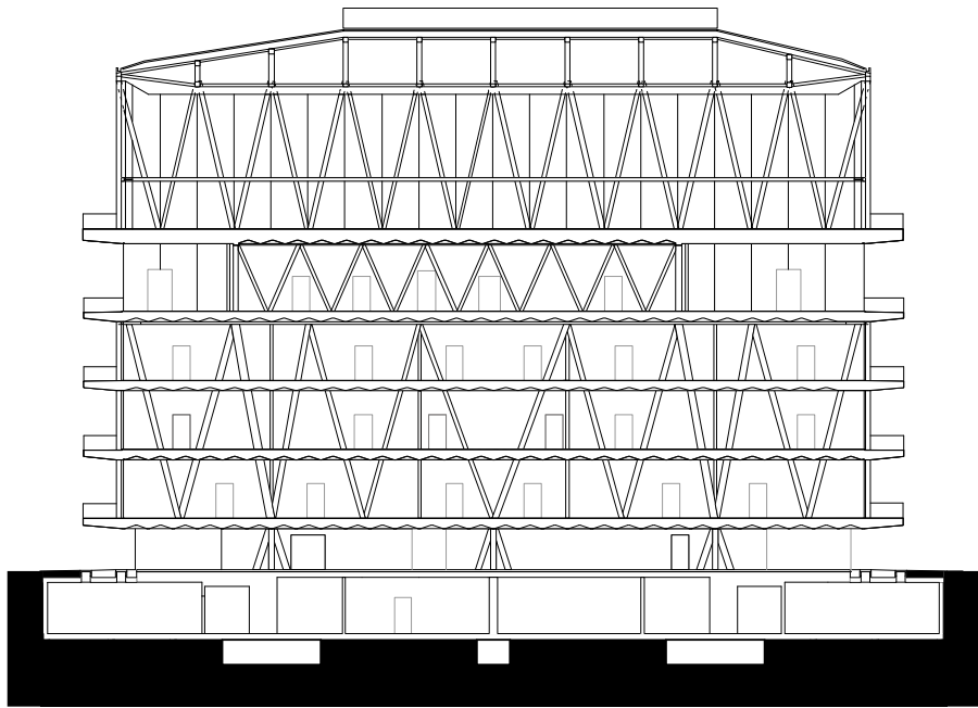
Leutschenbach, Logitudinal Section
