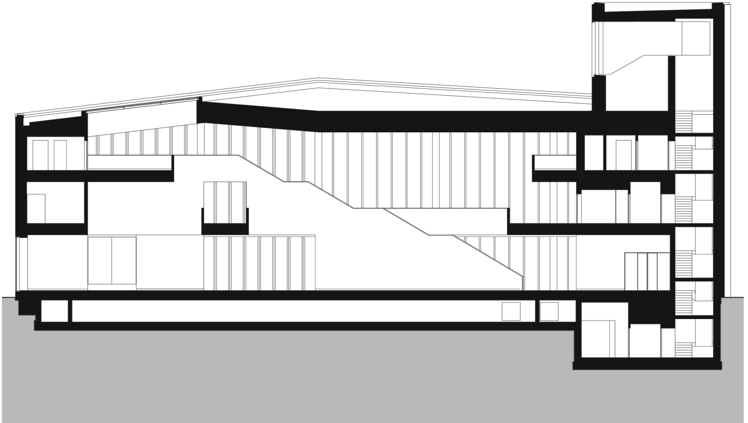
section DD
